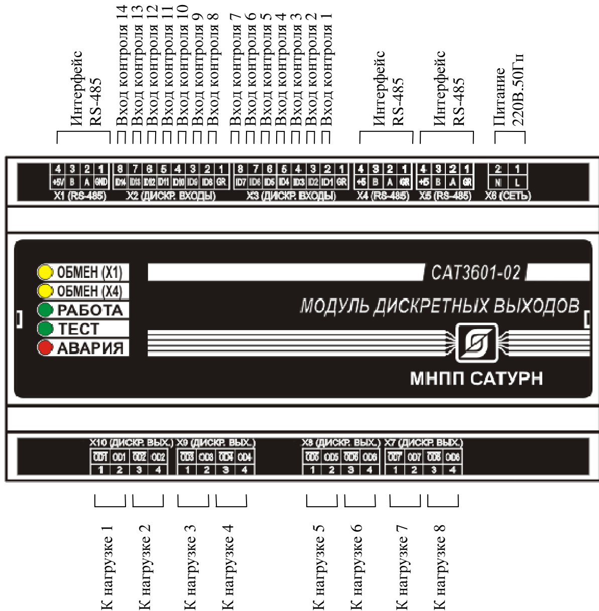
Рисунок 4 - Расположение разъемов на плате САТ3601-02
