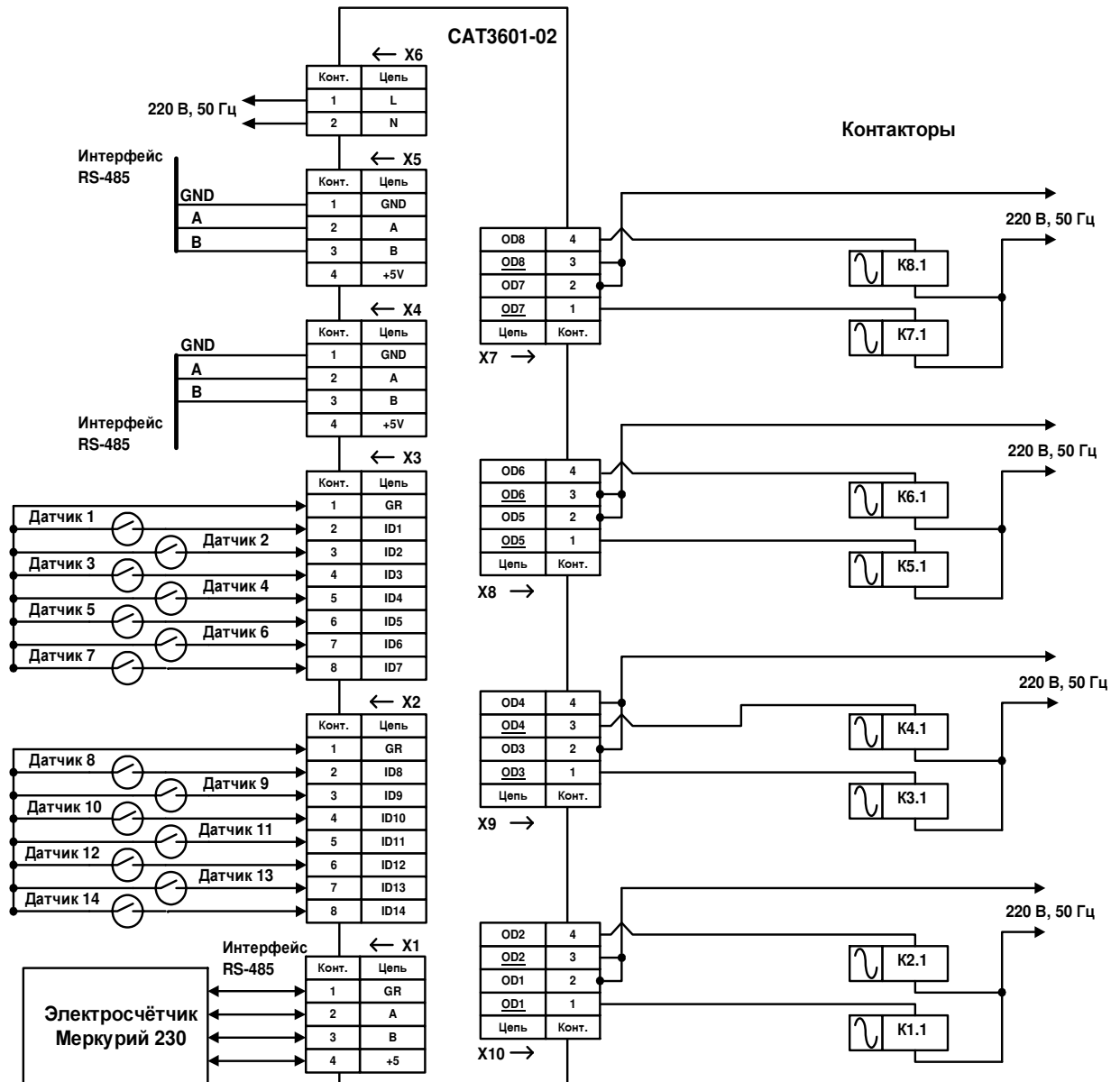
Рисунок 5 - Электрическая принципиальная схема подключения САТ3601-02 (типовая)
