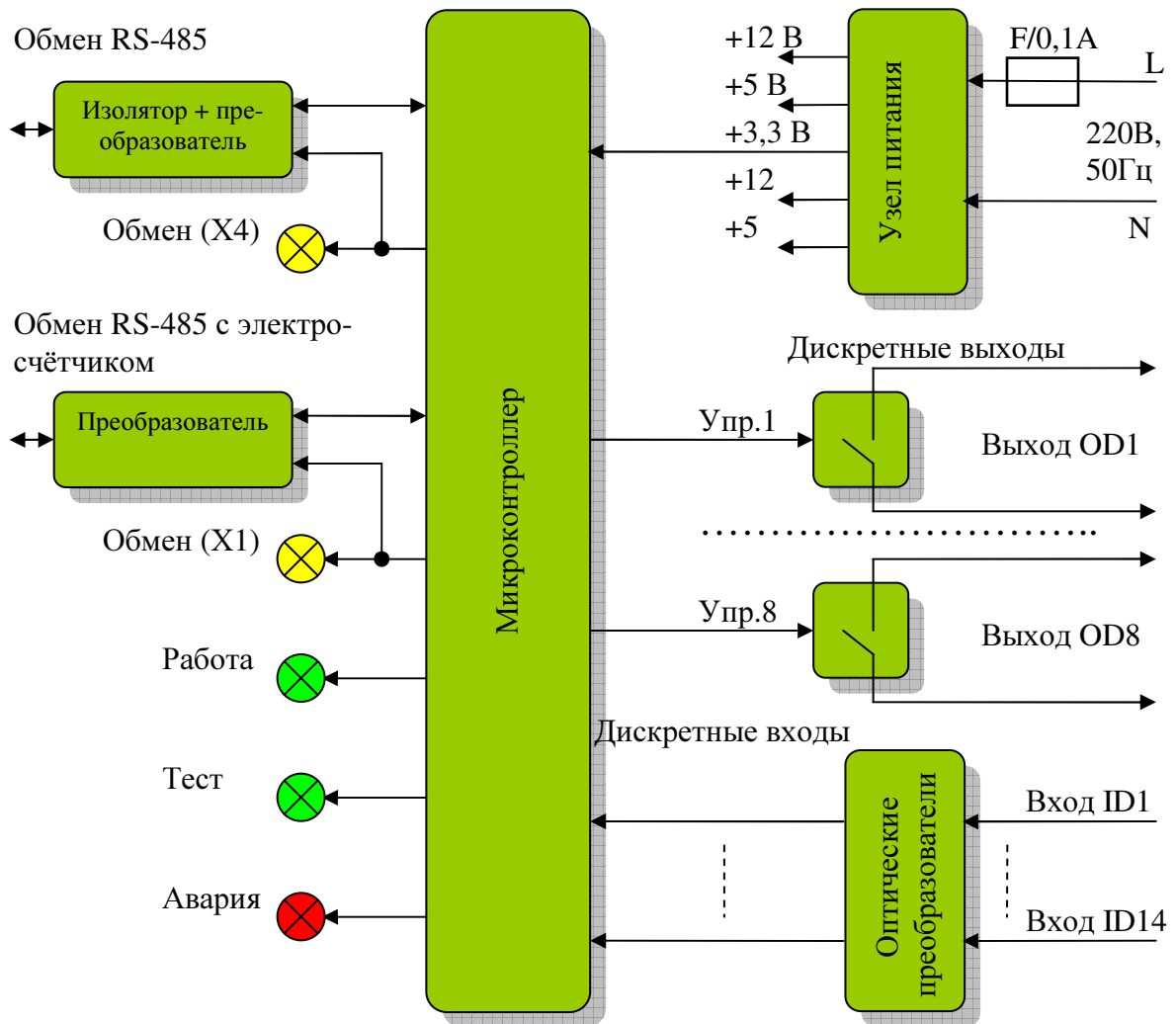
Рисунок 2 - Структурная схема САТ3601-02
